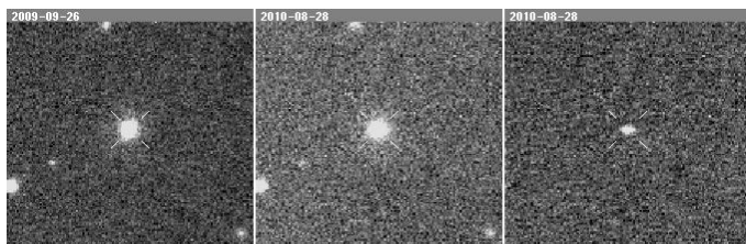
Supernova 2010hv
