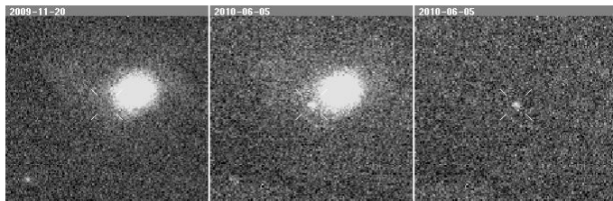
Supernova 2010ec
