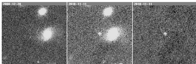
Supernova 2010jq
