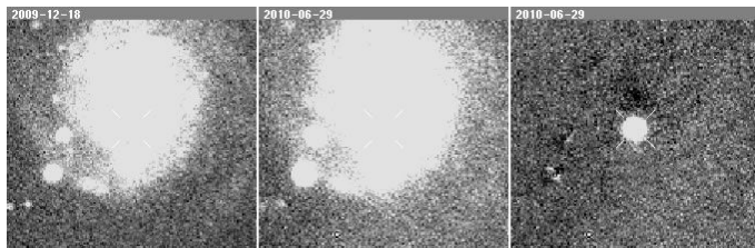
Supernova 2010ev
