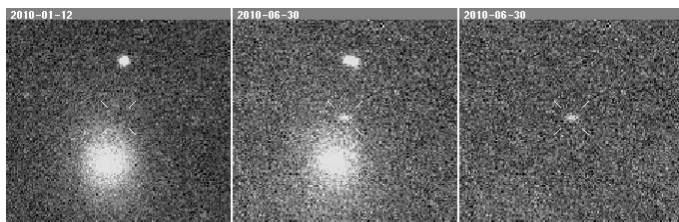
Supernova 2010ey
