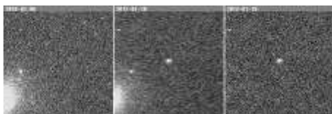
Supernova 2012H
