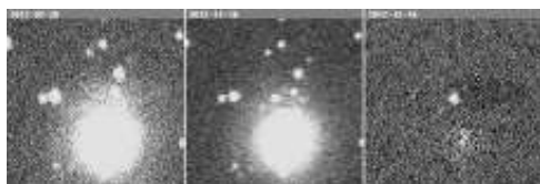
Supernova 2012hv
