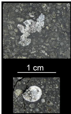
Calcium Aluminum Inclusions (CAIs) en Allende.
