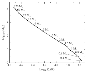
Modelo de ZAMS ( fig. reproducida de Carroll & Ostlie)
