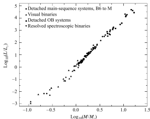
Observaciones de luminosidades estelares ( fig. reproducida de Carroll & Ostlie)
