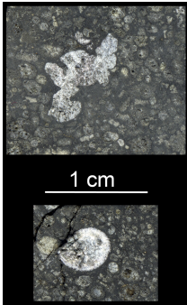
Calcium Aluminum Inclusions (CAIs) en Allende.
