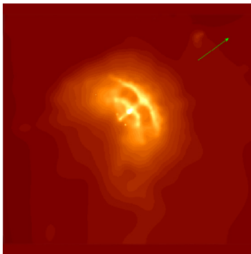
Vela X
