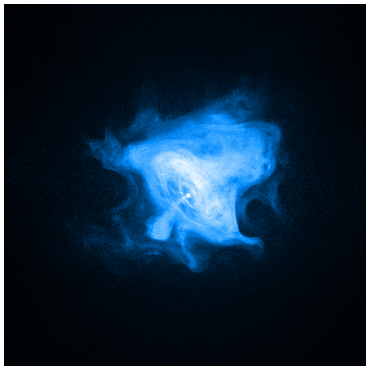
Cangrejo
