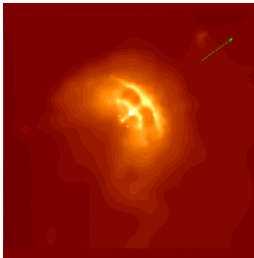
Vela X
